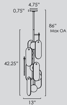
SM24827 • Vertical Pendant
