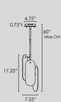
SM24811 • Stem Hung Pendant
