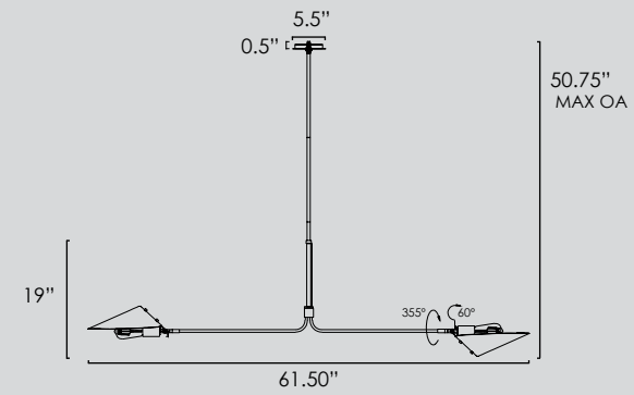
SM81802 • Linear Pendant
