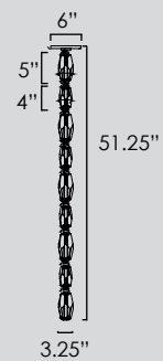
SM24864 • Single Pendant
