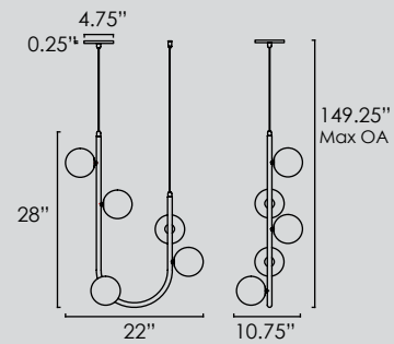
SM24905 • Cord Hung Pendant
