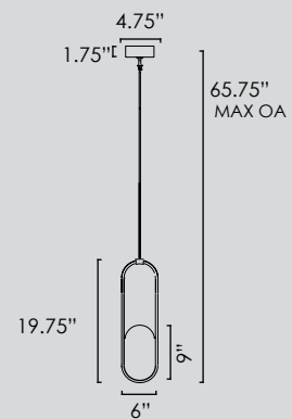
SM24881 • Mini Pendant
