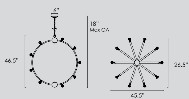
SM23776 • Large Pendant
