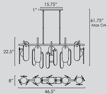
SM24825 • Linear Pendant
