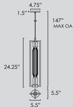
SM24843 • Single Pendant
