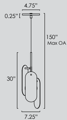
SM24812 • Cord Hung Pendant
