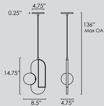
SM24602 • Side-Light Pendant
