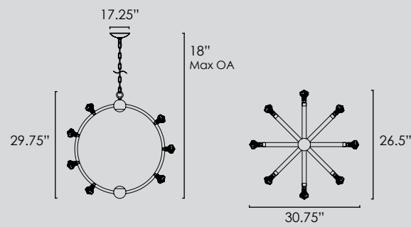
SM23774 • Medium Pendant
