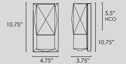
SM23642 • ADA Sconce
