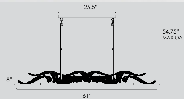
SM23819 • Linear Pendant
