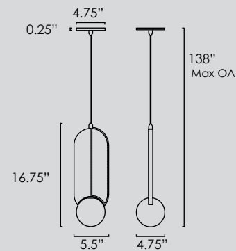
SM24603 • Down-Light Pendant
