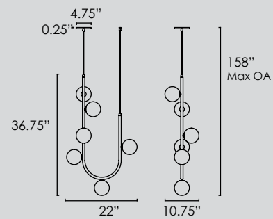
SM24906 • Cord Hung Pendant
