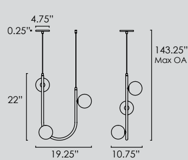
SM24903 • Cord Hung Pendant
