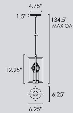
SM24841 • Mini Pendant
