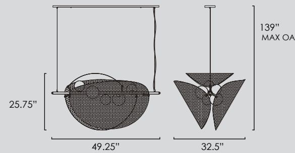
SM32305 • Linear Pendant
